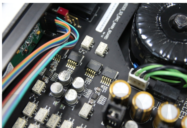
S3耳擴是採用每聲道各兩顆Ti LME49600作平衡輸出，在32歐姆之下可輸出2,000mW。
